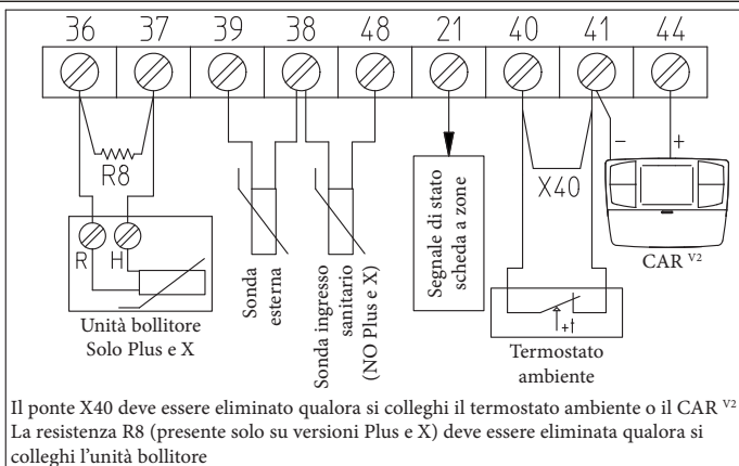
Cronotermostato digitale On/Off
